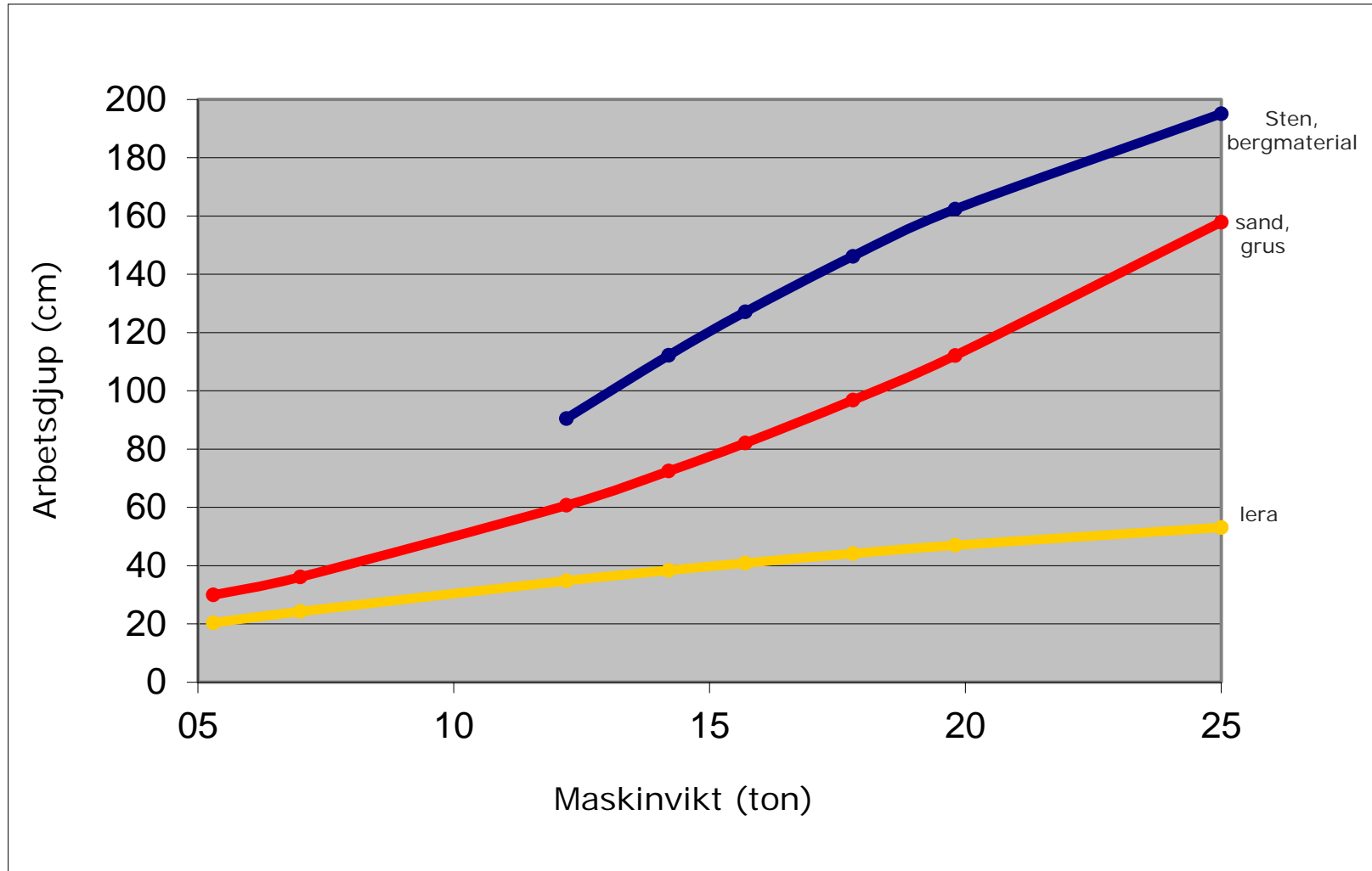
Översikt arbetsdjup i relation med maskinvikt
